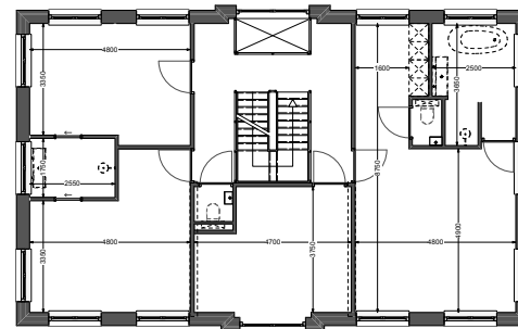
1E VERDIEPING
