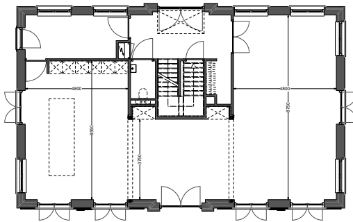
BEGANE GROND
