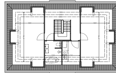
2E VERDIEPING
