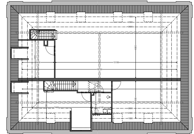
2E VERDIEPING
