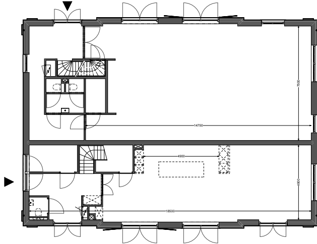
BEGANE GROND
