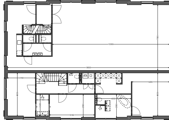
1E VERDIEPING
