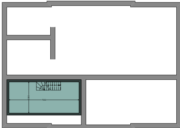
KELDER
